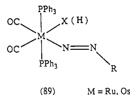
(89) M = Ru, Os
